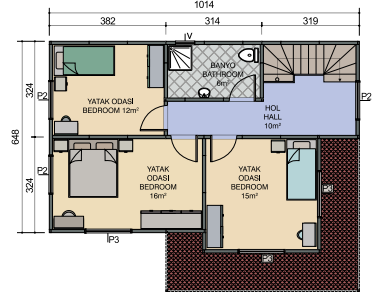
1. Kat Planı First Floor Plan 64m 2
