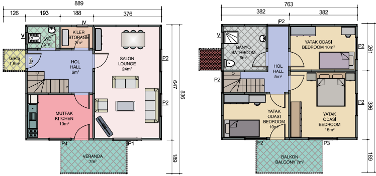
Zemin Kat Planı Ground Floor Plan 49m^2 + 9m^2 = 58m^2
