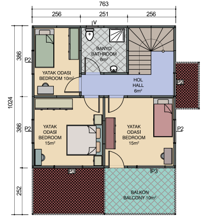
1. Kat Planı First Floor Plan 58m 2 + 10m 2 = 68m 2
