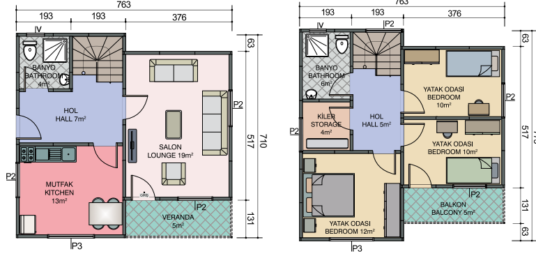
Zemin Kat Planı Ground Floor Plan 46m^2 + 5m^2 = 51m^2
