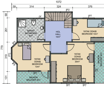
1. Kat Planı First Floor Plan 66m^2 + 11m^2 = 77m^2
