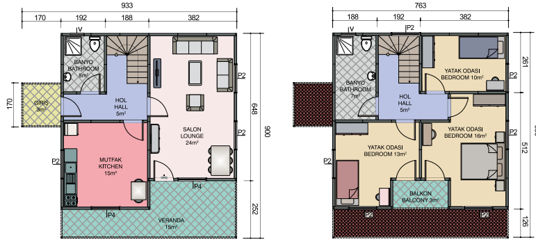
Zemin Kat Planı Ground Floor Plan 54m^2 + 18m^2 = 72m^2
